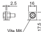
■ Type 4 Flag M6
